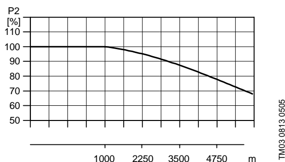
Fig. 1 Relación entre el rendimiento del motor ( P_2 ) y la altitud.
