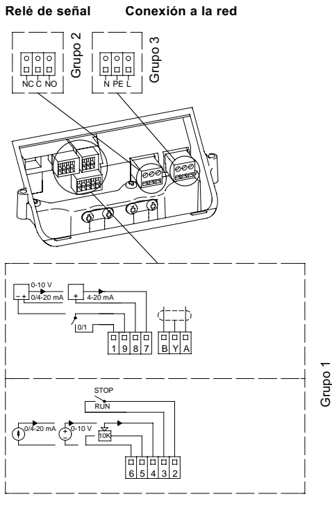
Fig. 27 Esquema de conexiones eléctricas, bombas TPE monofásicas
