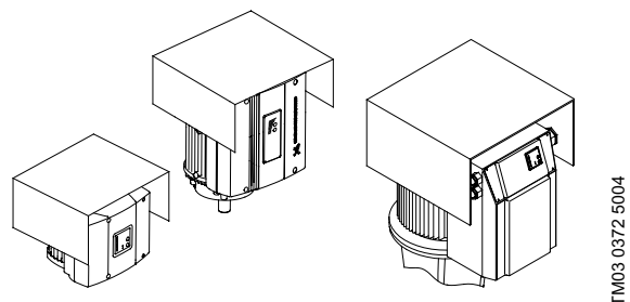
Fig. 19 Motores MGE y MMGE con cubierta de condensación
