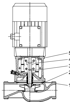
Fig. 3 Plano seccionado de TP Serie 100 (con conexión de unión)
