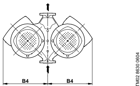
Fig. 24 Posiciones de las cajas de conexiones de bombas TPED
