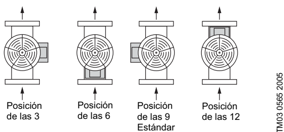
Fig. 23 Posiciones posibles de la caja de conexiones
