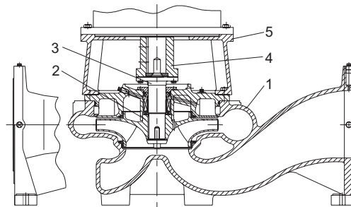
Fig. 8 Plano seccionado de TP Serie 400
