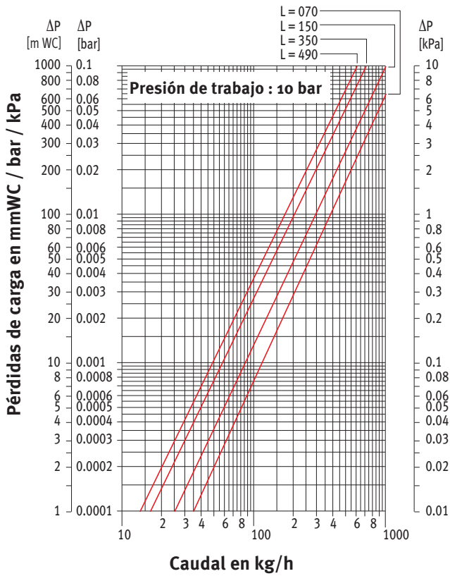
PÉRDIDA DE CARGA TIPO 09 CONEXIONES OPUESTAS
