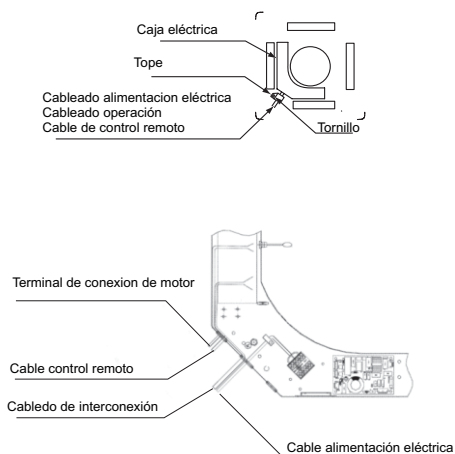
Fig. 7.1 Conexión cableado eléctrico unidad interior
