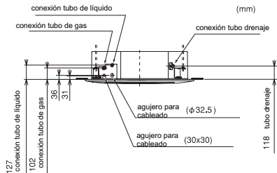
Fig.3.6 Unidad interior y panel frontal
