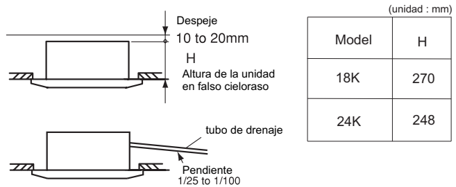
Fig. 3.2 Lugar de instalación de unidad interior
