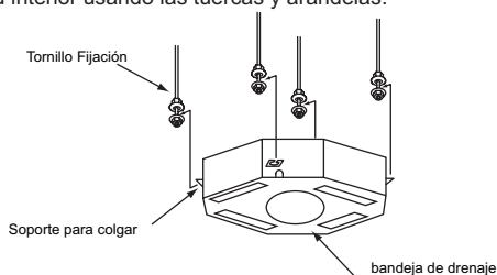
Fig. 3.8 Montando la unidad interior
