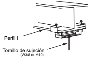
Fig. 3. 4. Montaje de tornillos de sujeción
