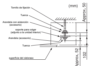
Fig. 3. 7 Montando tuercas y arandelas
