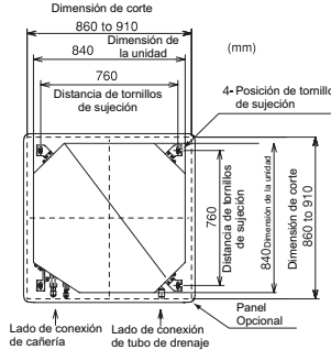
Fig. 3. 3 Apertura de cieloraso y colocación tornillos de sujeción
