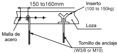
Fig. 3. 4. Montaje de tornillos de sujeción
