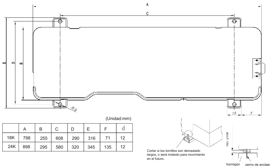
Fig. 4.2 instalación de los pernos de anclaje
