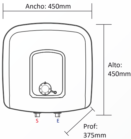
Dimensiones HT-30
