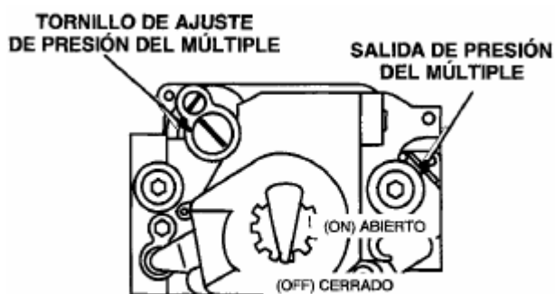
VÁLVULA DE GAS MOSTRADA EN POSICIÓN OFF
