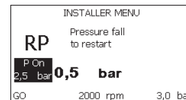
Kuva 17: Uudelleenkäynnistysarvojen asetus
