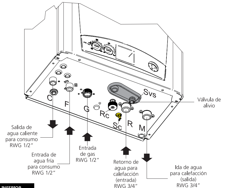
VISTA INFERIOR
